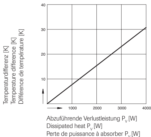
Leistungsdiagramm/Performance diagram/Diagramme de puissance
