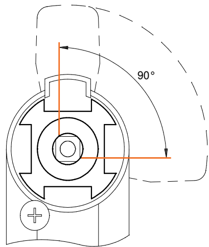
Türscharniere rechts Door hinged right charnière droite de porte
