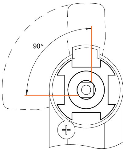
Anschlag einstellen Cam position fixer la butée
